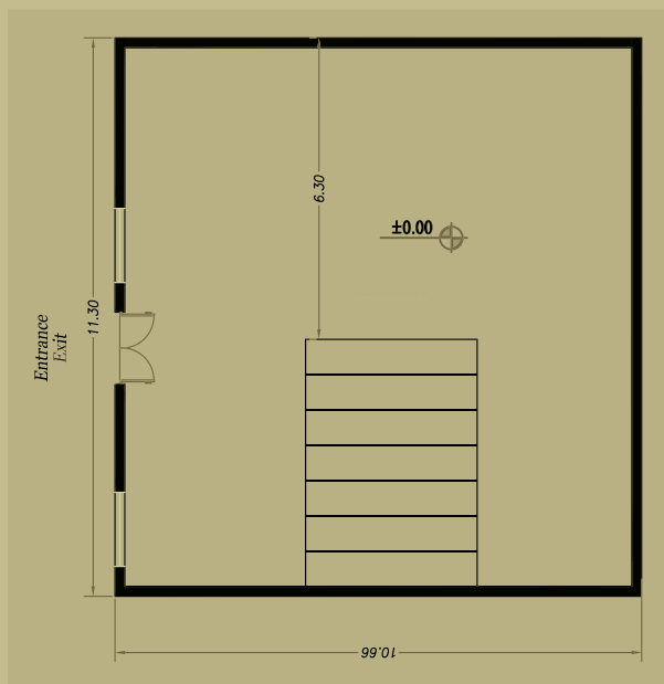
نقشه ترسیمی
