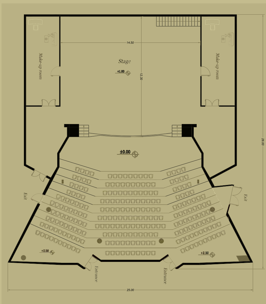
نقشه ترسیمی
