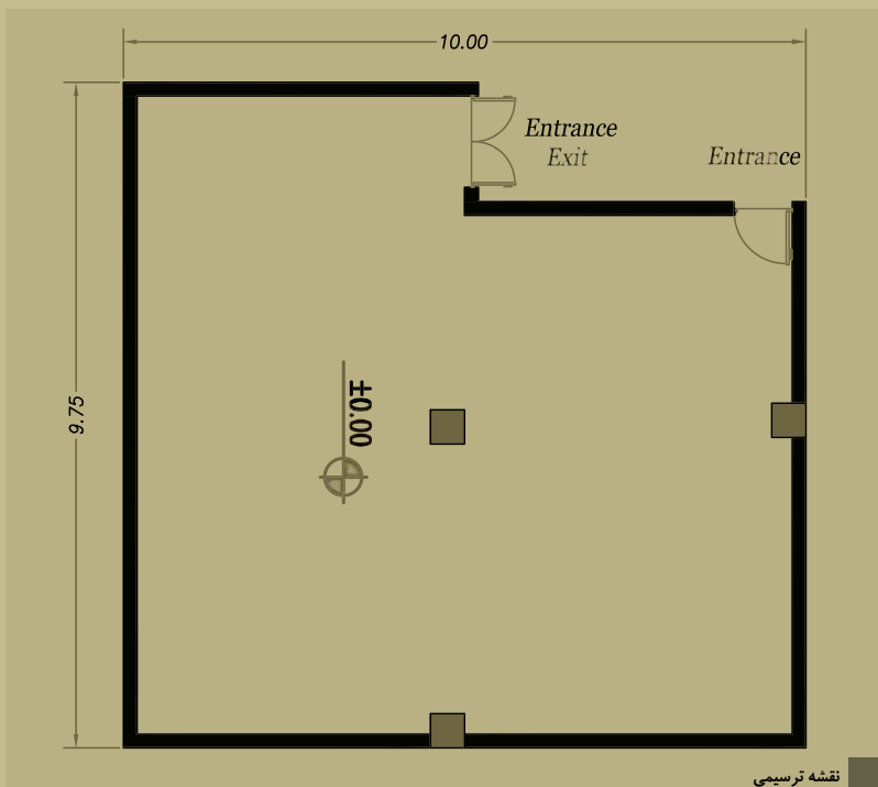
نقشه ترسیمی
