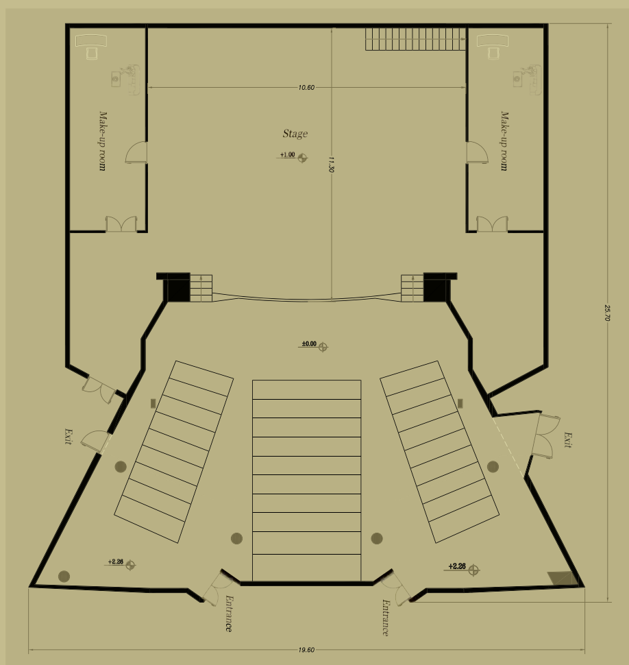
نقشه ترسیمی
