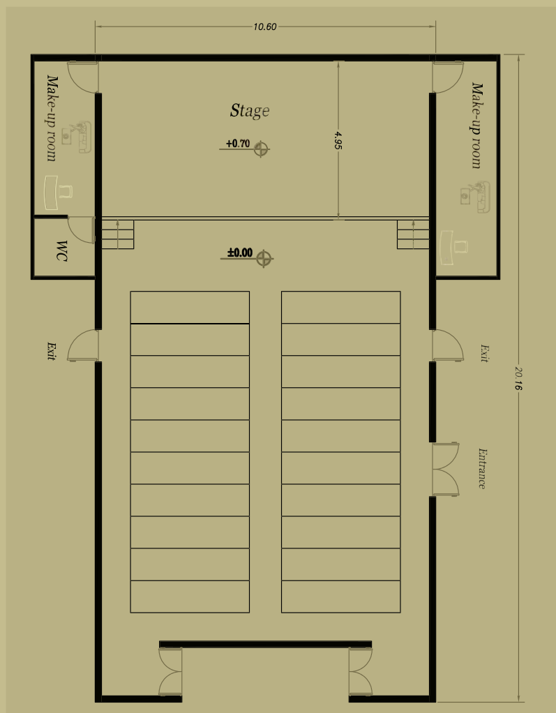
نقشه ترسیمی
