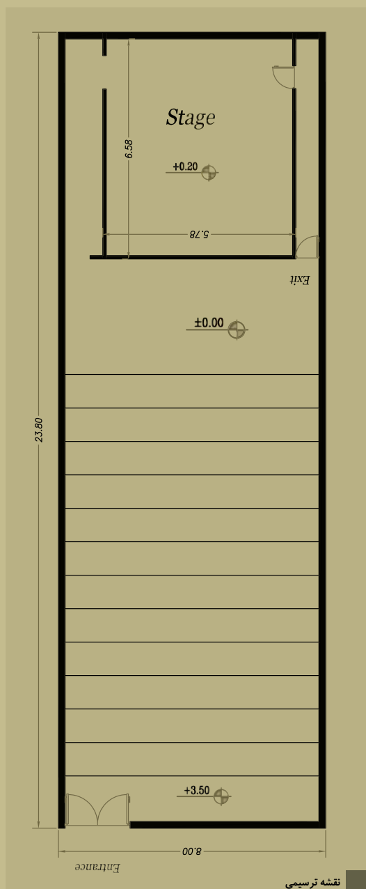
نقشه ترسیمی
